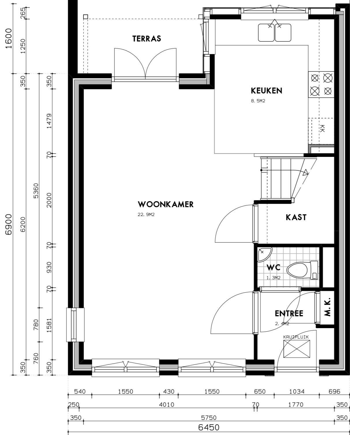
BEGANE GROND
