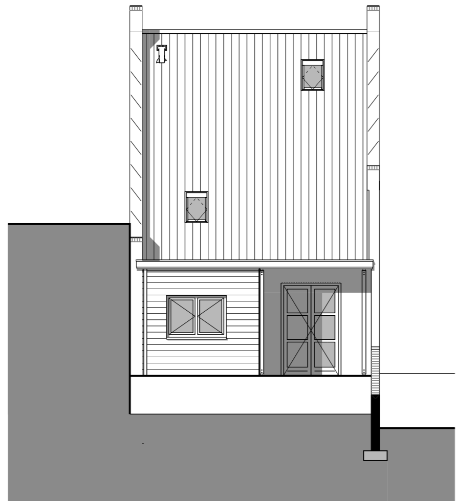
ACHTERGEVEL
