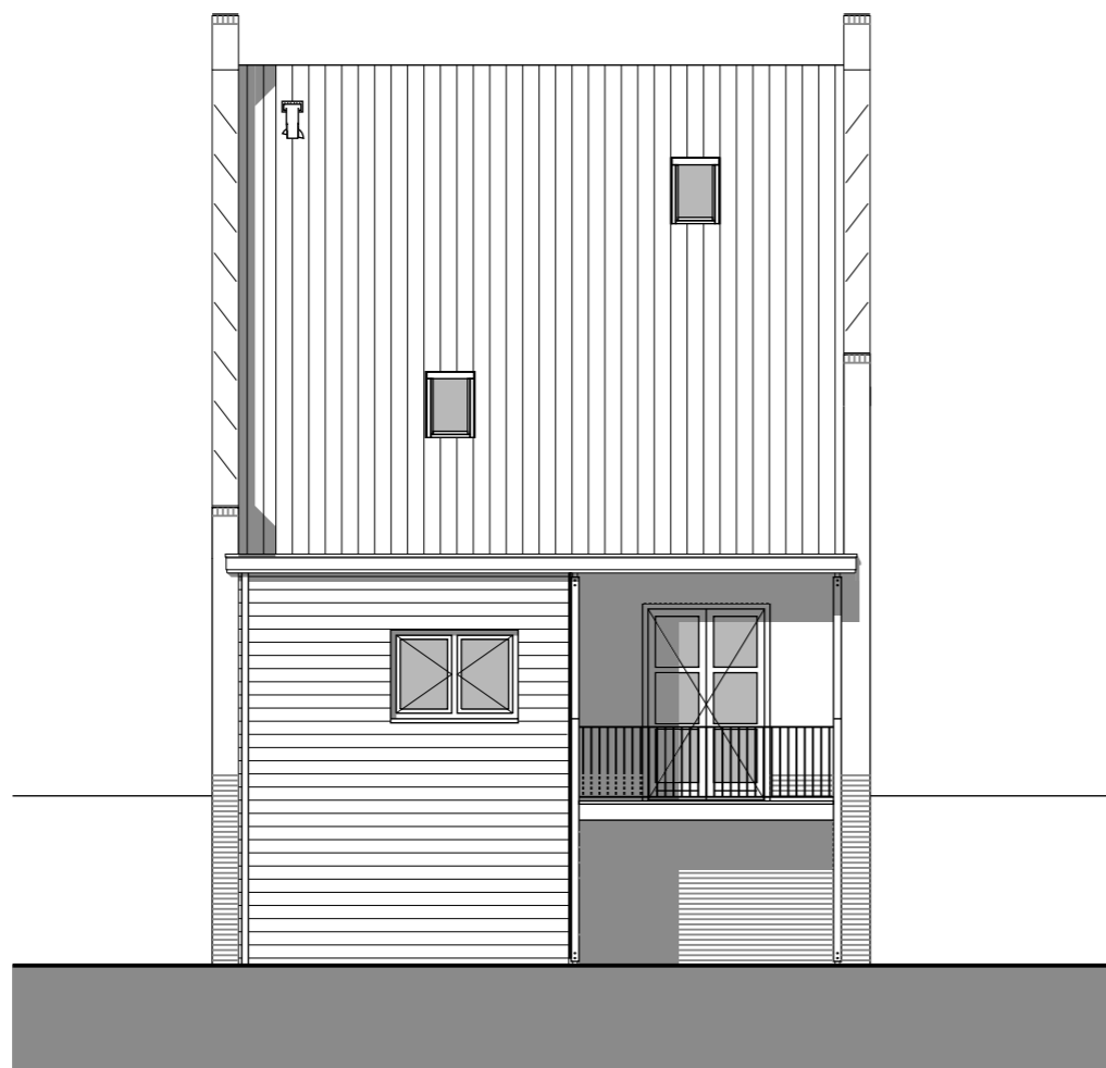
ACHTERGEVEL
