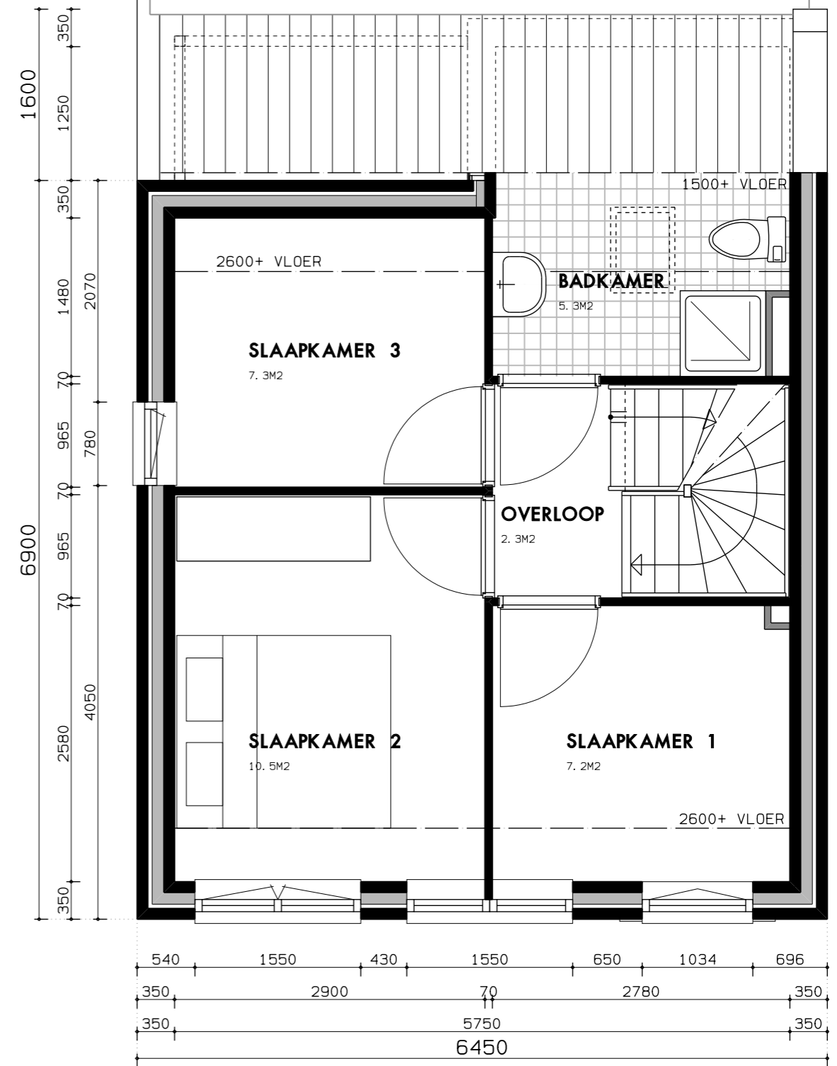
EERSTE VERDIEPING
