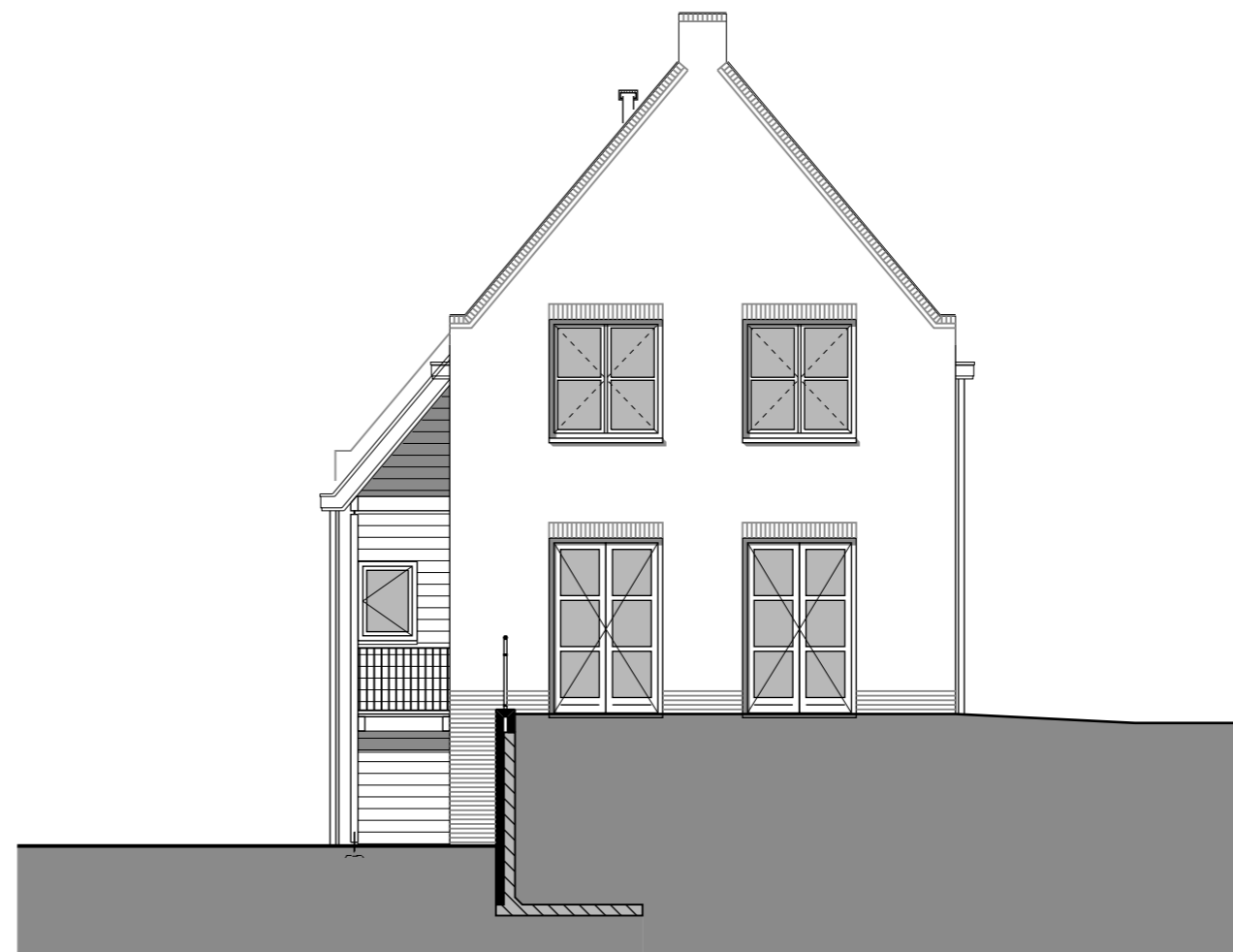
LINKER ZIJGEVEL
